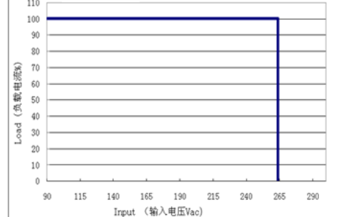
图 3-2-1 负载-输入电压降额曲线 (负载电流—输入电压降额曲线)
