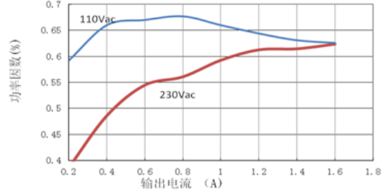
图 1-4-2 功率因数vs输出电流 at 48V, typ.
