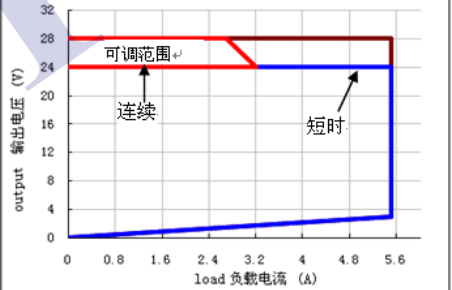
图 3-1-1 输出 V-I 曲线 (输出负载特性曲线)
