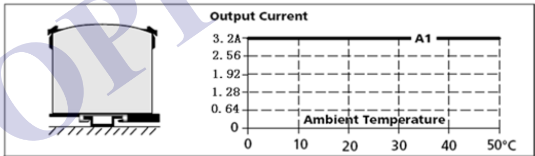
图 7-3-1 安装方向 C (桌面安装) (24V 输出电压)
