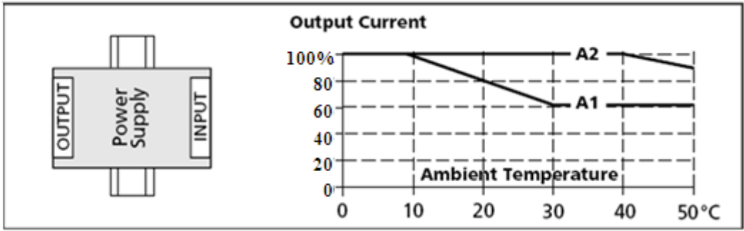
图 7-5 安装方向 E (水平安装方向) (12V 输出电压)
