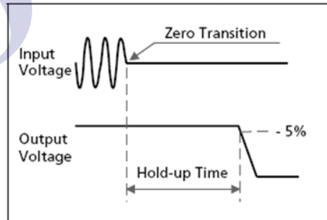
图 3-4 关机曲线
