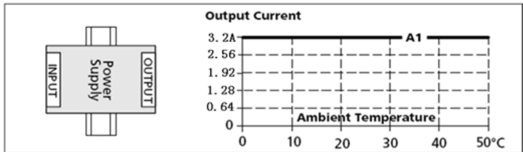
图 7-4-1 安装方向 D (水平安装方向) (24V 输出电压)
