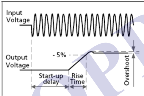
图 3-3 开机曲线
