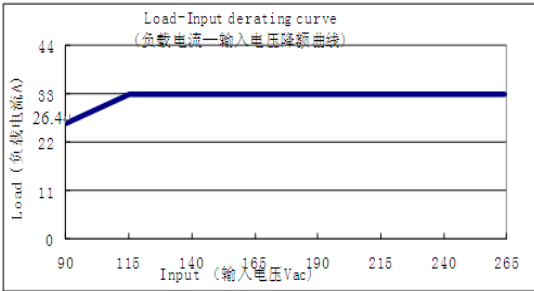
1. 负载电流—输入电压降额曲线 (24V 输出电压) :
