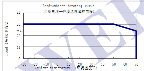
2. 负载电流—环境温度降额曲线 (24V 输出电压) :
