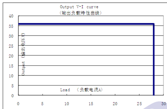
输出特性曲线图(36V 输出电压) :
