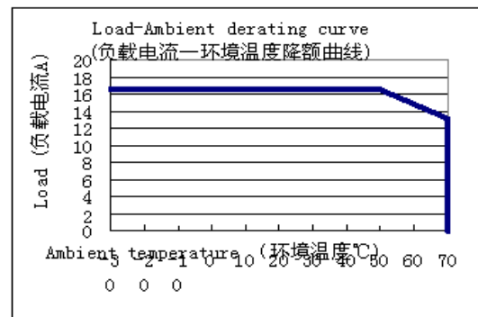
6. 负载电流—环境温度降额曲线 (48V 输出电压) :
