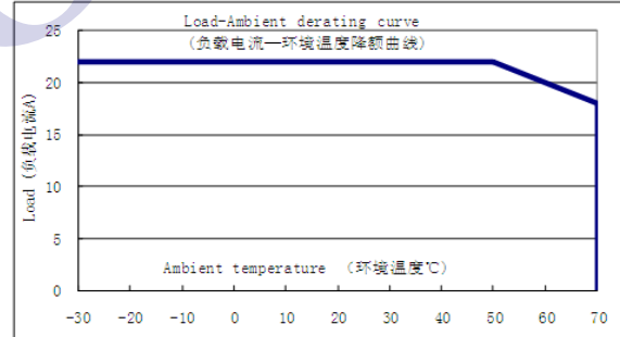
4. 负载电流—环境温度降额曲线 (36V 输出电压) :
