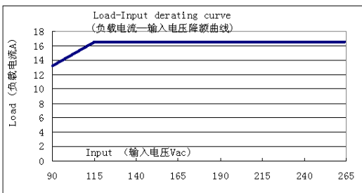
5. 负载电流—输入电压降额曲线 (48V 输出电压) :
