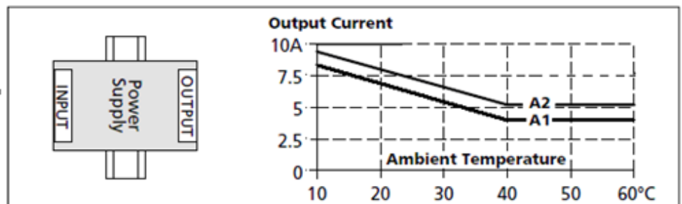
图 7-4-1 安装方向 D (水平安装方向) (36V 输出电压)
