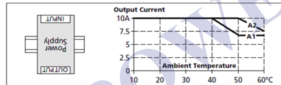
图 7-2-1 安装方向 B (倒转方向) (36V 输出电压)
