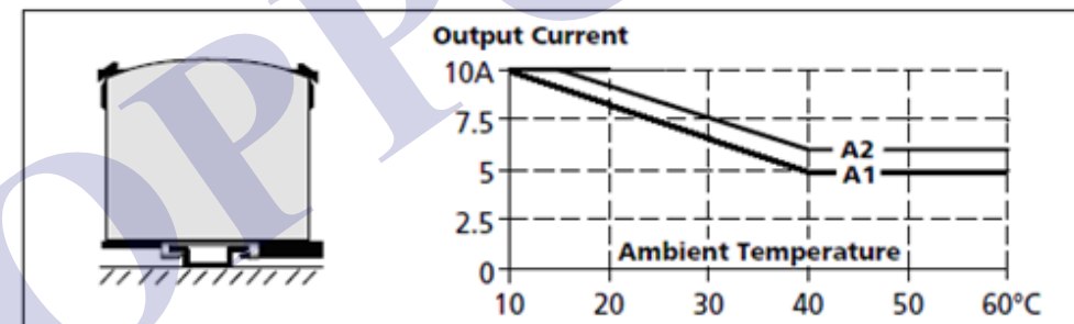
图 7-3-1 安装方向 C (桌面安装) (36V 输出电压)
