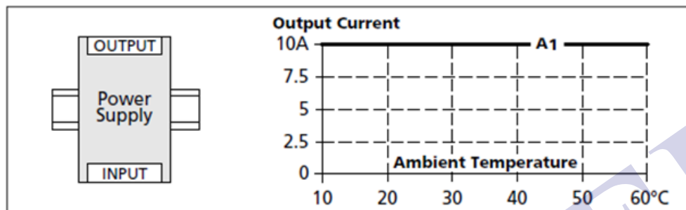
图 7-1-1 安装方向 A (标准安装方向) (36V 输出电压)
