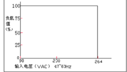
输出负载降额与输入电压关系
