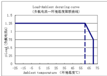
降额曲线图 (12V 输出电压):
